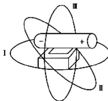
图 B.1 X 射线管组装体泄漏辐射 三圆周检测位置示意图
